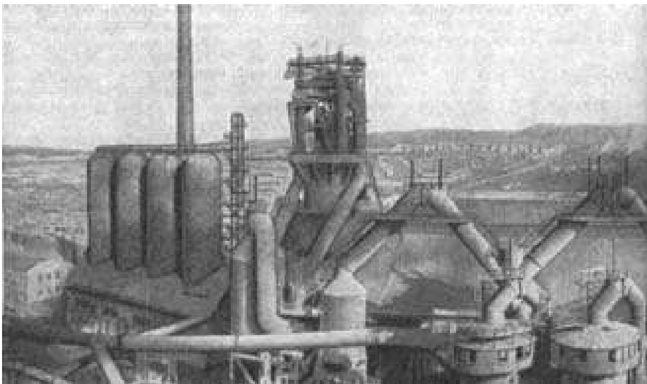
Доменный цех Кузнецкого металлургического завода. Фотография. 1934 г.
