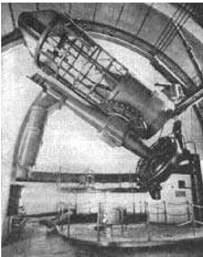
82-дюймовый телескоп Мак-Дональда на Маунт Лок в Техасе. Фотография. 1939 г.
